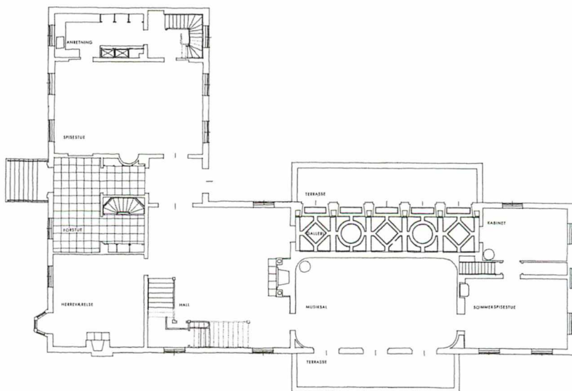
Terkel Hjejle og Niels Rosenkjær: Egebækgård. Plan af hovedbygningen, 1916.
