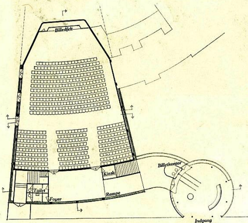
Plan af 1. Etage
