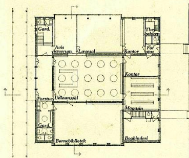
Plan af Bibliotekets Stueetage
