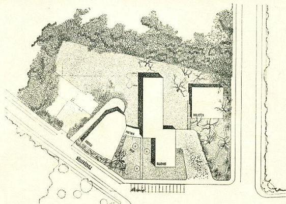
Arne Jacobsen og Flemming Lassen: Raadhus for Søllerød Kommune Bygningen, set fra Kongevejen. Beliggenhedsplan med Angivelse af det projekterede Bibliotek og Biograf 1:2000
